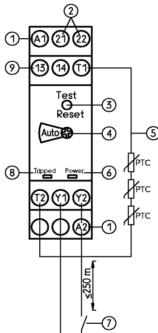
Abbildung 10: Kaltleiter-Auslösegerät
