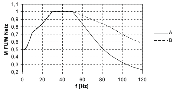
Diagramm 5: Baugröße 180-200
