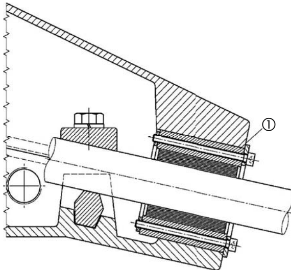
Abbildung 7: Kabeleinführung
