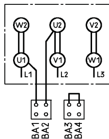
Δ-Schaltung
