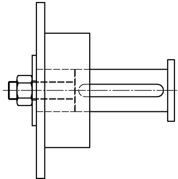
Abbildung 4: Befestigung von Riemenscheibe oder Kupplung
