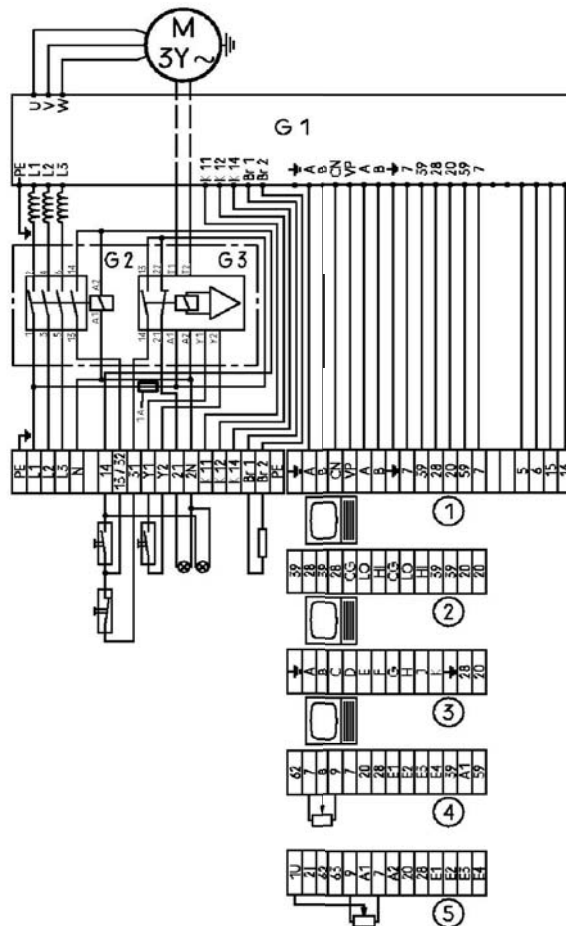
Abbildung 12: Übersichtsschaltbild Kompaktantrieb mit Schütz und Kaltleiter-Auslösegerät und interner Spannungsversorgung für TN-Netz.
